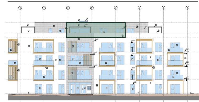
Pohľad ZÁPADNÝ
